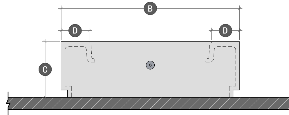
CY.1.3 SIDE ELEVATION SCALE: 1" = 1' - 3"
